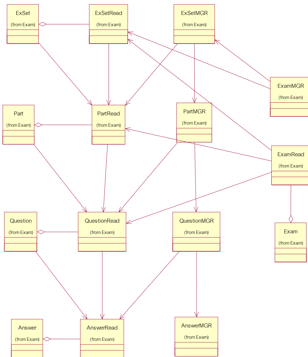
รูปที่ 7-82 รูปแสดง Class Diagram ของส่วนการสร้างแบบทดสอบ
