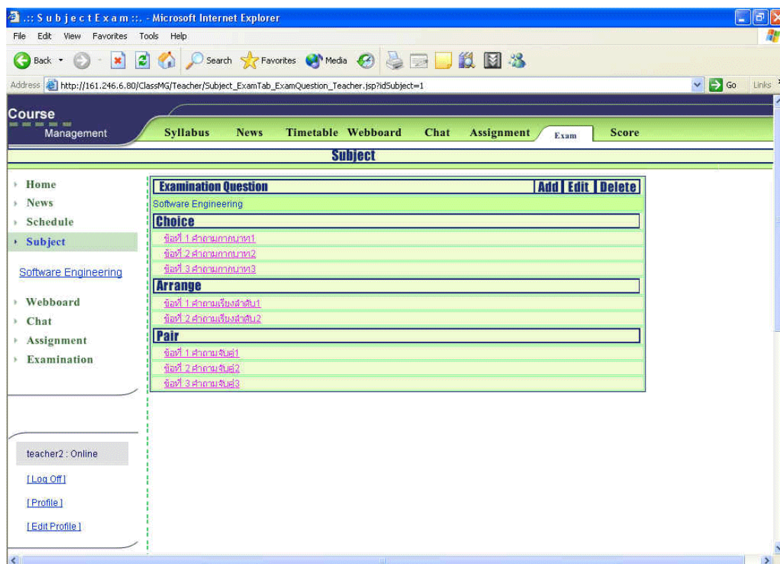
รูปที่ 7-64 รูปแสดง user interface ของส่วนแสดงข้อสอบทั้งหมดของอาจารย์
