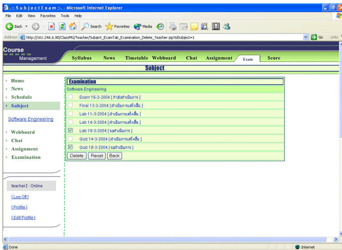
รูปที่ 7-81 รูปแสดง user interface ของส่วนลบกำหนดการสอบของอาจารย์
