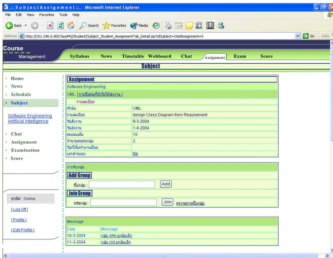
รูปที่ 7-53 รูปแสดง user interface ของส่วน Assignment ของนักศึกษา
