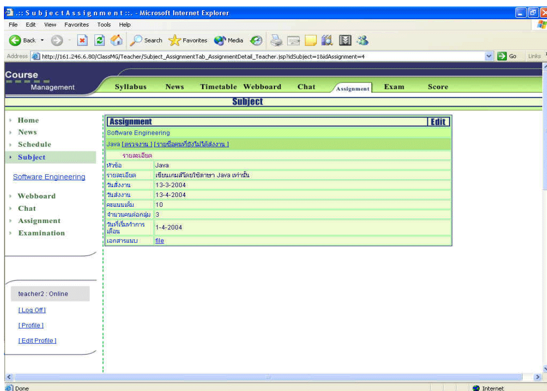
รูปที่ 7-54 รูปแสดง user interface ของส่วนรายละเอียด Assignment ของอาจารย์
