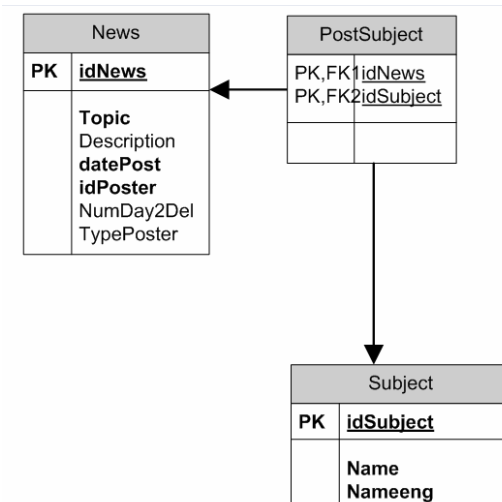
รูปที่ 7-25 รูปแสดงรายละเอียดโครงสร้างตารางของส่วนข่าวสาร
