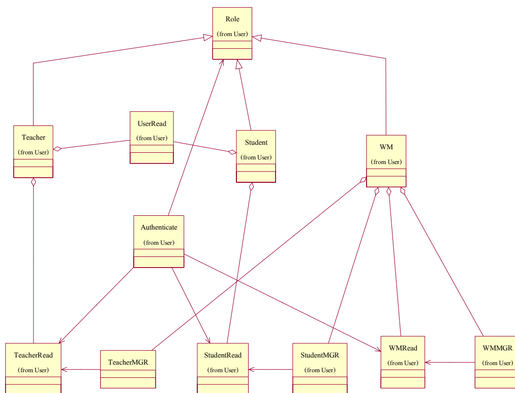
รูปที่ 7-10 รูปแสดง Class Diagram ของส่วนเข้าสู่ระบบและข้อมูลส่วนตัว
