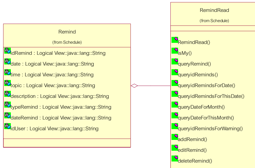
รูปที่ 7-90 รูปแสดง Class Diagram ของส่วนกำหนดการ
