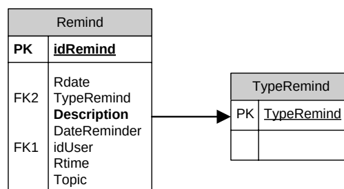
รูปที่ 7-92 รูปแสดงรายละเอียดโครงสร้างตาราง ของส่วนกำหนดการ
