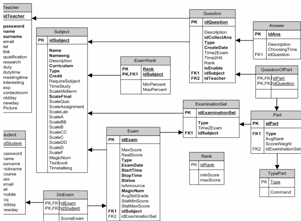
รูปที่ 7-84 รูปแสดงรายละเอียดโครงสร้างตารางของส่วนการสร้างแบบทดสอบ
