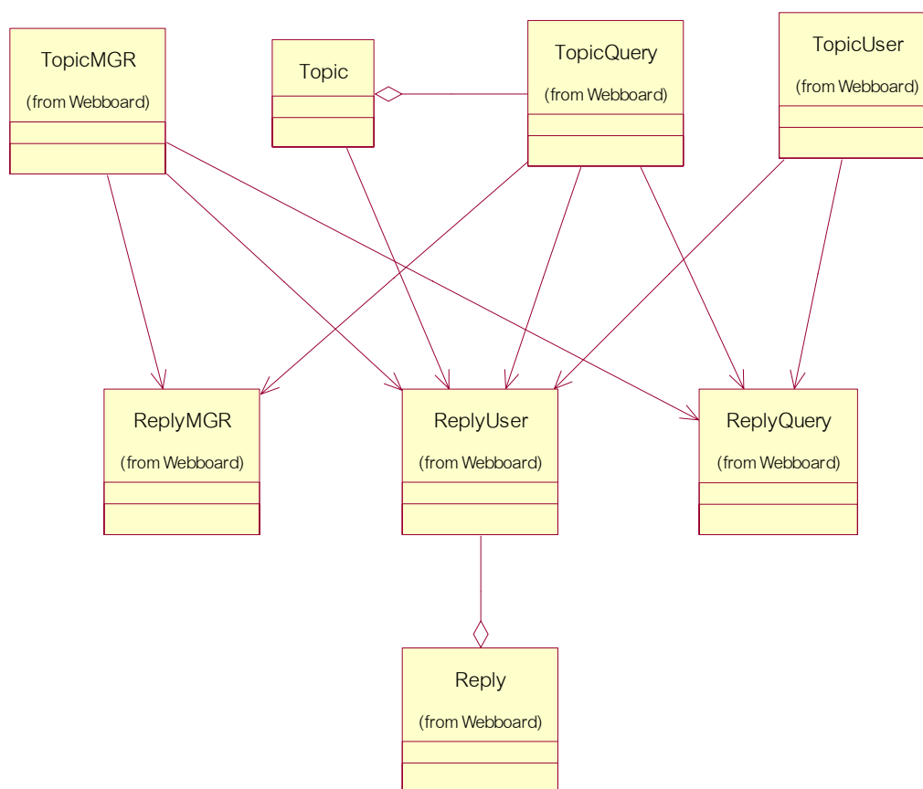
รูปที่ 7-47 รูปแสดง Class Diagram ของส่วนเว็บบอร์ด
