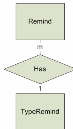
รูปที่ 7-91 รูปแสดง ER Diagram ของส่วนกำหนดการ
