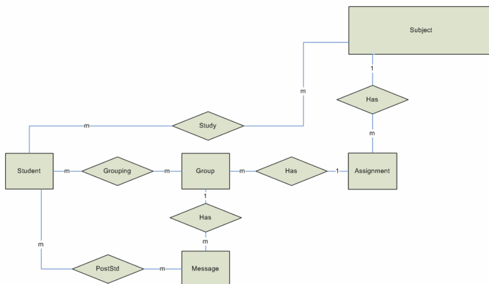
รูปที่ 7-59 รูปแสดง ER Diagram ของส่วน Assignment
