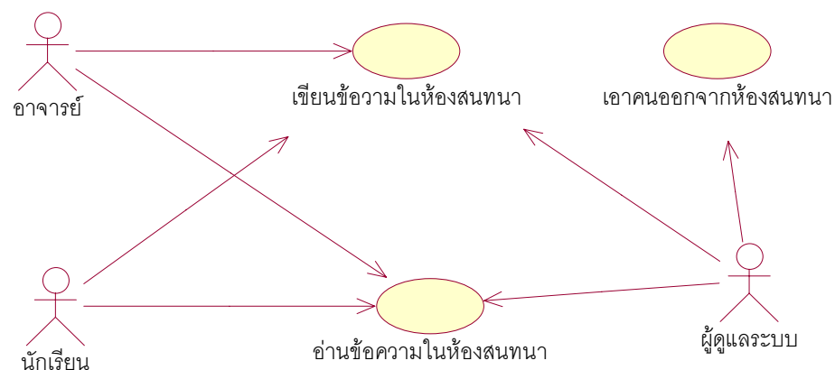
รูปที่ 7-50 รูปแสดง user case diagram ของส่วนห้องสนทนา
