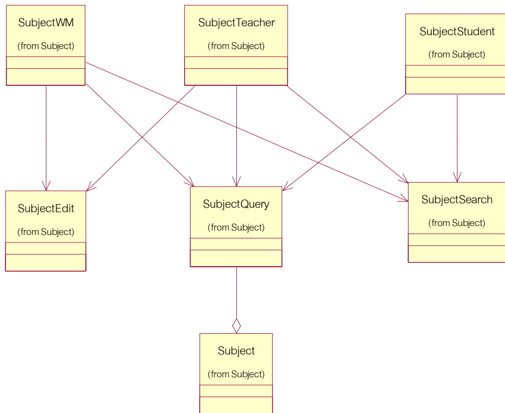
รูปที่ 7-39 รูปแสดง Class Diagram ของส่วนรายวิชา
