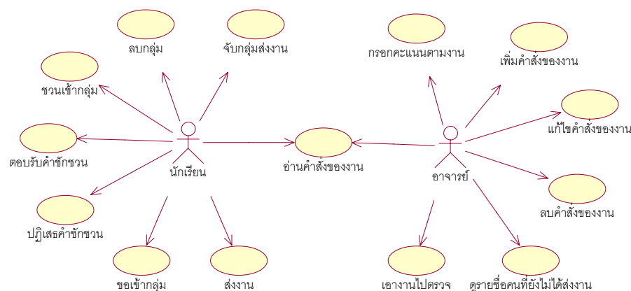
รูปที่ 7-52 รูปแสดง Use Case Diagram ของส่วน Assignment
