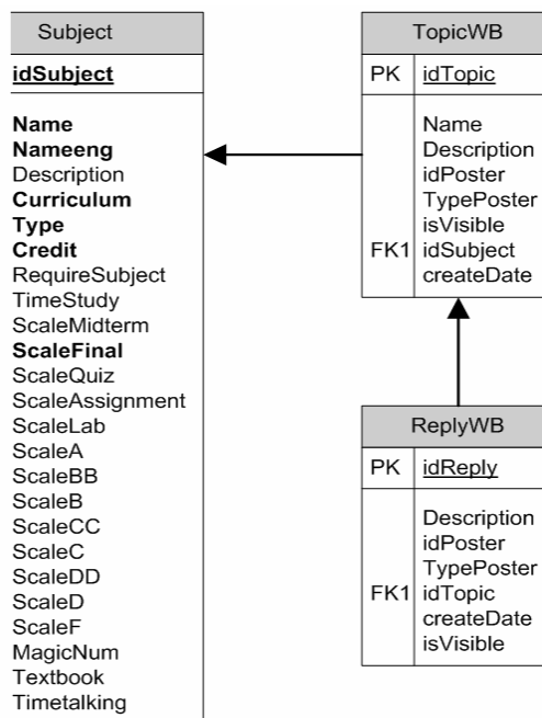
รูปที่ 7-49 รูปแสดงรายละเอียดโครงสร้างตารางของส่วนเว็บบอร์ด
