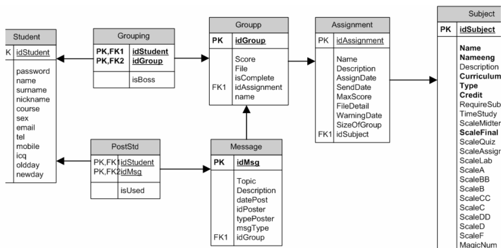
รูปที่ 7-60 รูปแสดงรายละเอียดโครงสร้างตารางของส่วน Assignment
