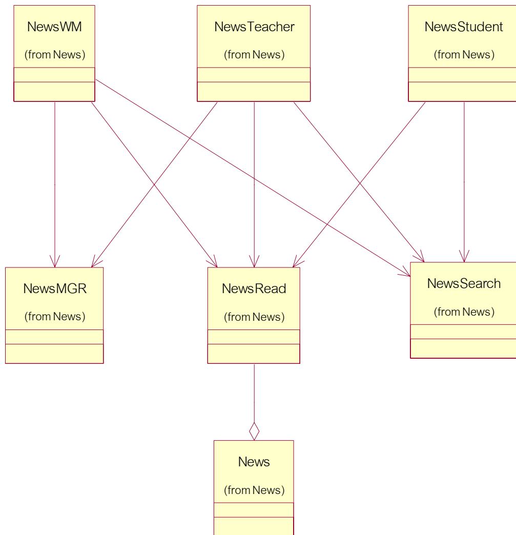
รูปที่ 7-23 รูปแสดง Class Diagram ส่วนของข่าวสาร
