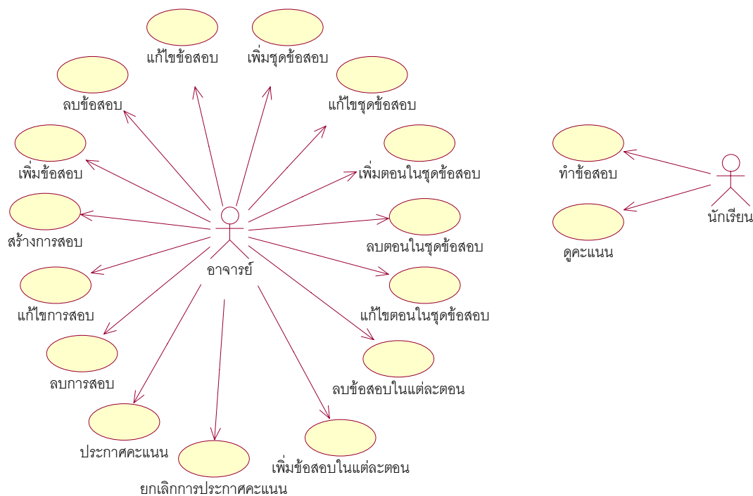
รูปที่ 7-61 รูปแสดง user case diagram ของส่วนสร้างแบบทดสอบ
