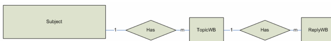
รูปที่ 7-48 รูปแสดง ER s Diagram ของส่วนเว็บบอร์ด
