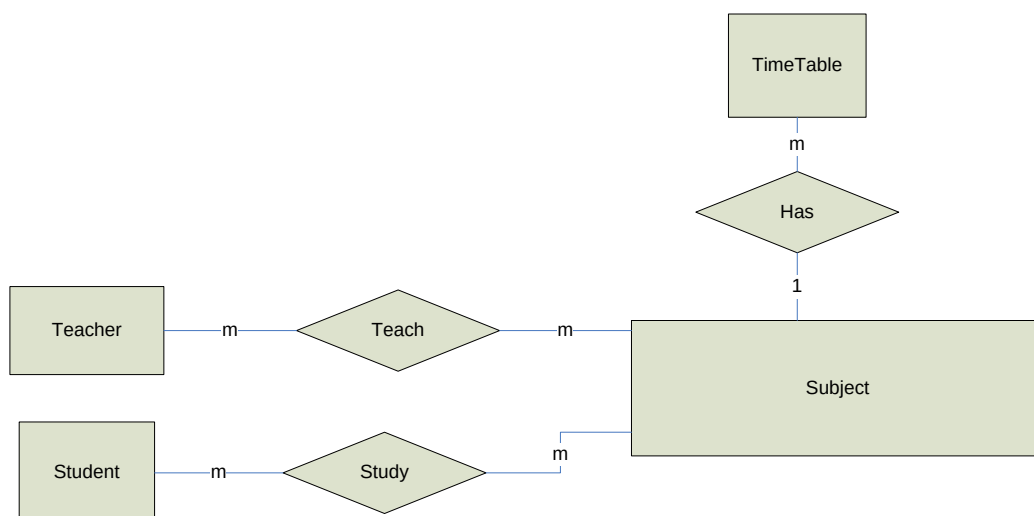
รูปที่ 7-40 รูปแสดง ER Diagram ของส่วนรายวิชา
