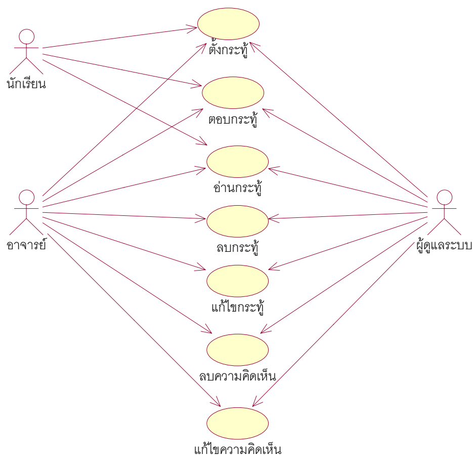
รูปที่ 7-42 รูปแสดง user case diagram ของส่วนเว็บบอร์ด
