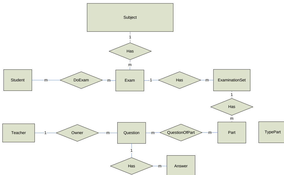
รูปที่ 7-83 รูปแสดง ER Diagram ของส่วนการสร้างแบบทดสอบ
