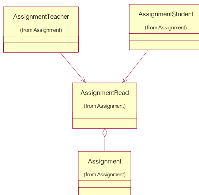
รูปที่ 7-58 รูปแสดง Class Diagram ของส่วน Assignment
