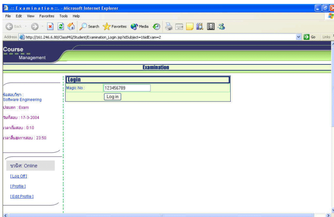
รูปที่ 7-62 รูปแสดง user interface ของส่วนใส่รหัสเพื่อทำข้อสอบ ของนักศึกษา
