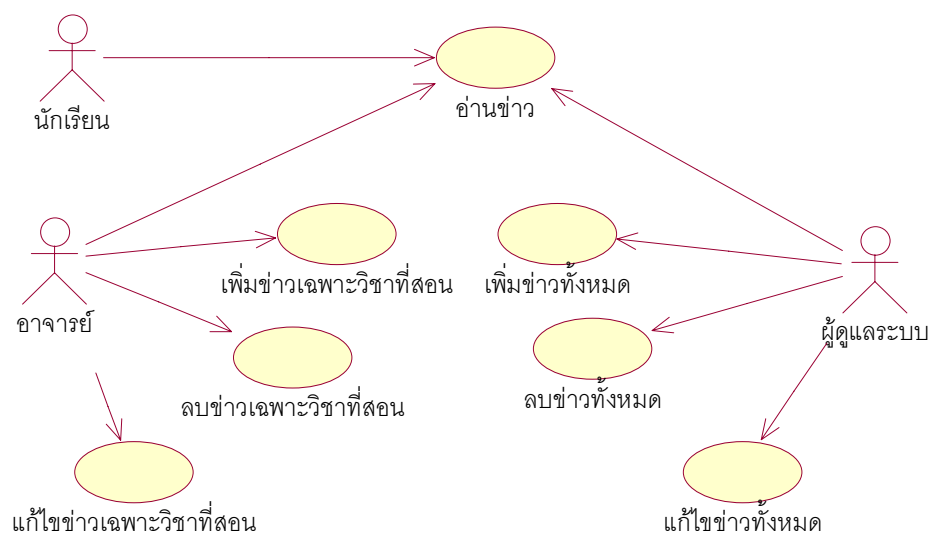
รูปที่ 7-13 รูปแสดง user case diagram ของส่วนข่าวสาร
