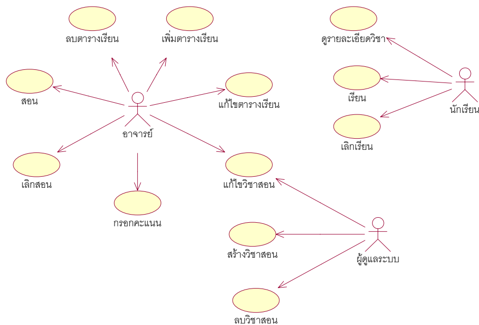
รูปที่ 7-26 รูปแสดง user case diagram ของส่วนรายวิชา
