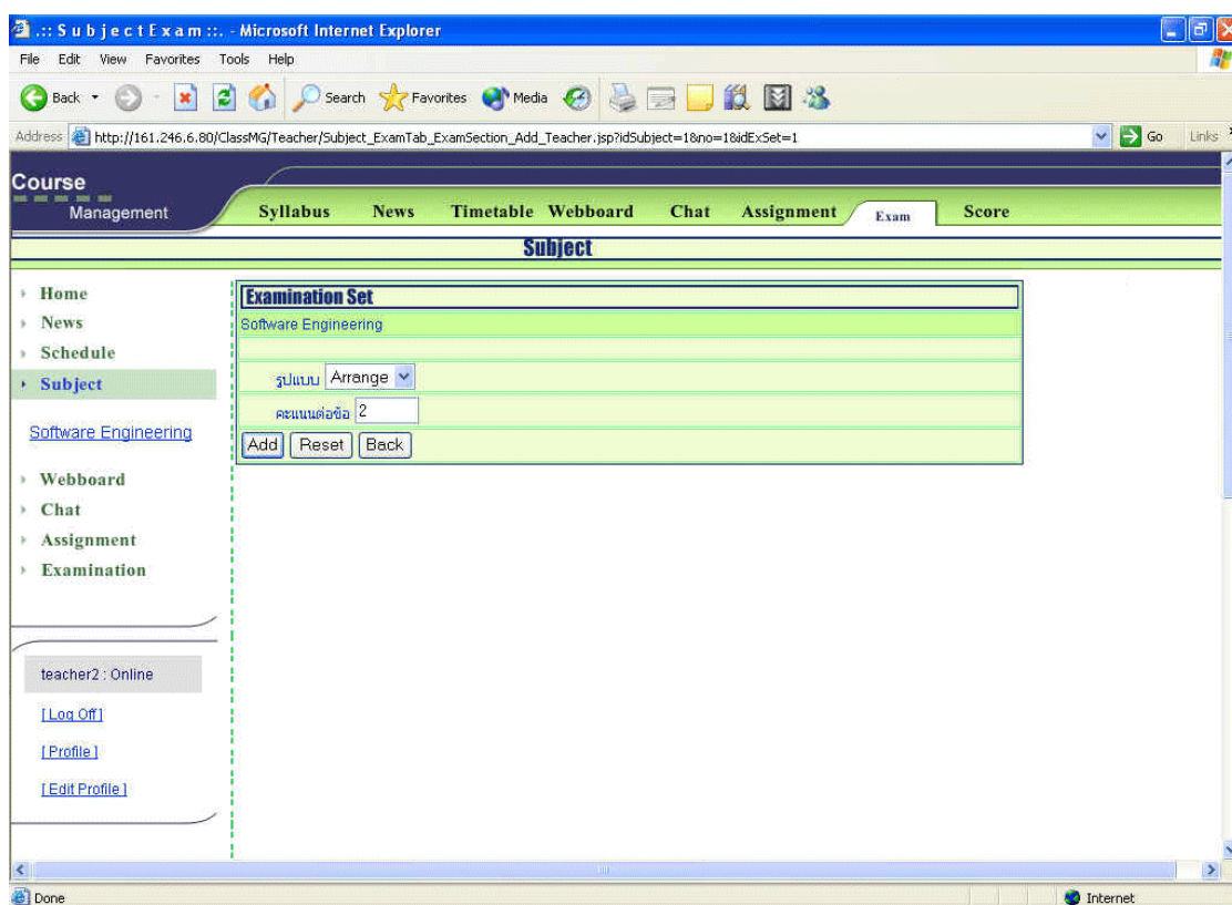
รูปที่ 7-72 รูปแสดง user interface ของส่วนเพิ่มตอนในชุดข้อสอบของอาจารย์
