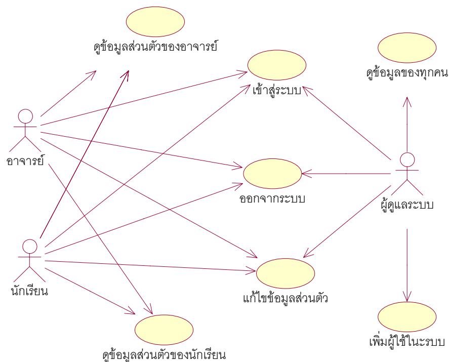
รูปที่ 7-1 รูปแสดง use case diagram ของส่วนเข้าสู่ระบบและข้อมูลส่วนตัว
