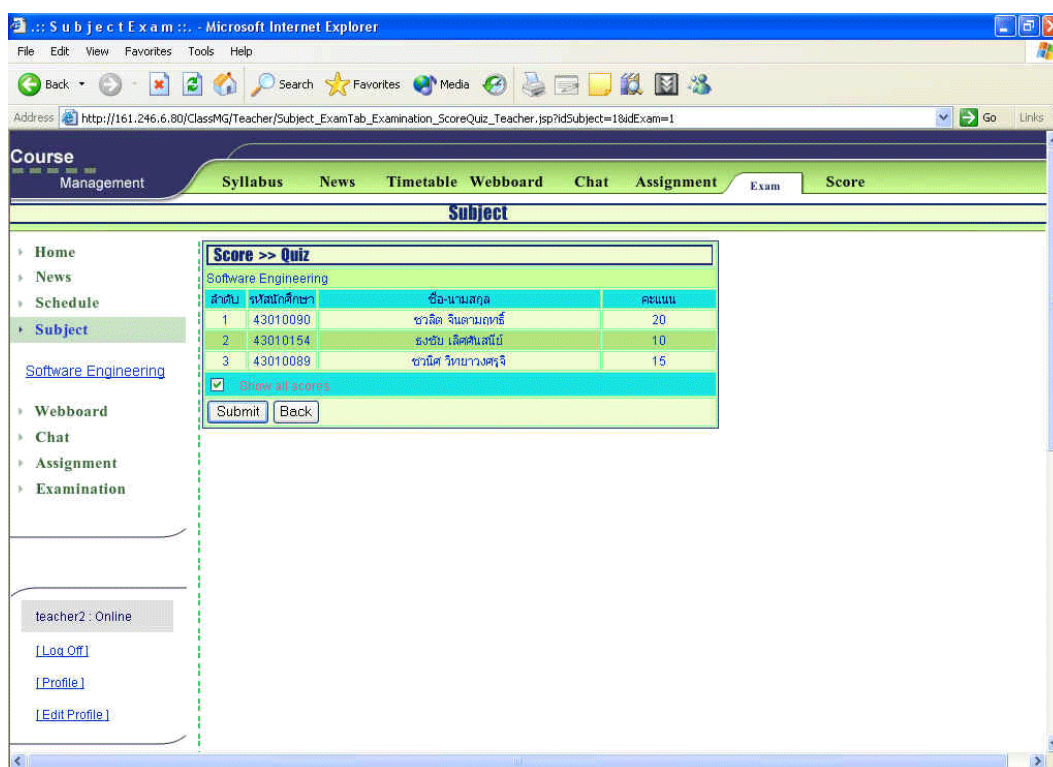
รูปที่ 7-37 รูปแสดง user interface ของส่วนจัดเก็บคะแนนที่เลือกให้แสดงคะแนนได้
