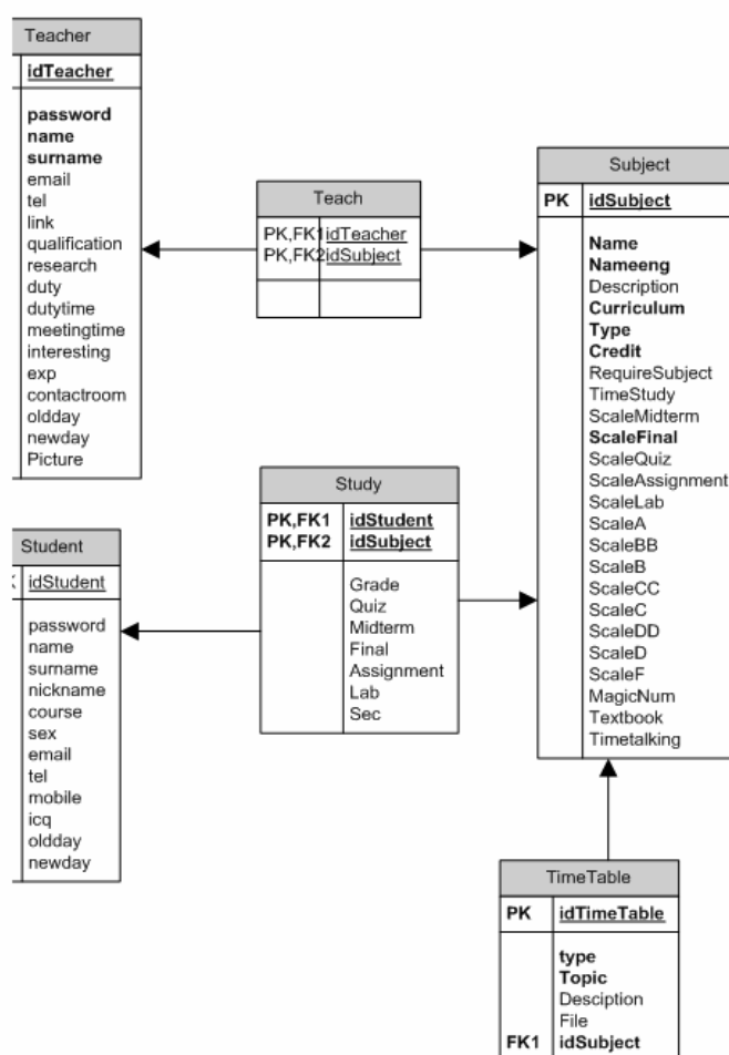
รูปที่ 7-41 รูปแสดงรายละเอียดโครงสร้างตารางของส่วนรายวิชา
